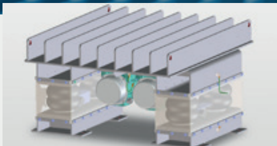
FÖRDERTECHNIK Vibriertisch
